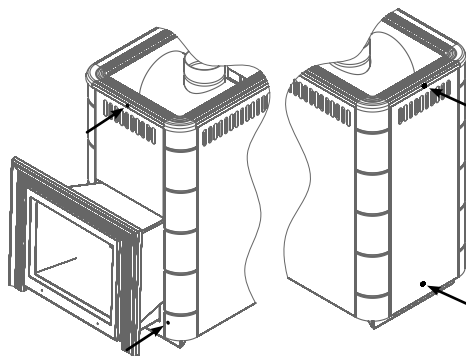
Рисунок 6. Винты для демонтажа конвектора печи «Ангара»
